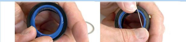
Abbildung 148: Abstreifer einlegen und befestigen
