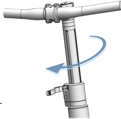
Abbildung 117: Beispiel All Up eingedreht
