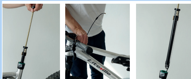
Abbildung 138: Kartusche herausziehen
