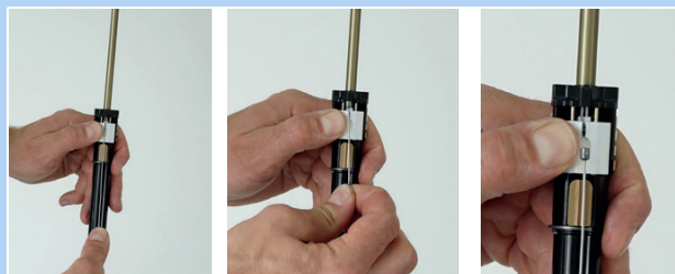
Abbildung 139: Seilzug aushängen
