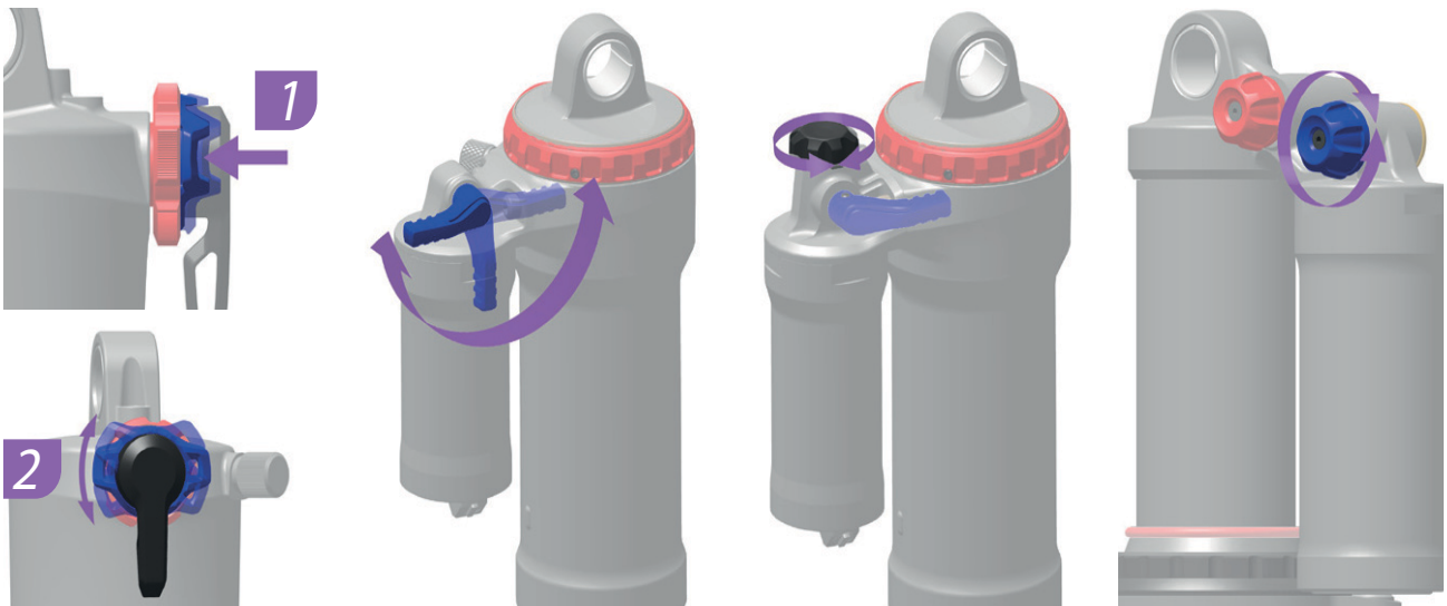
Abbildung 225: Lage und Form des Druckstufeneinstellers (blau) ist Modellabhängig
