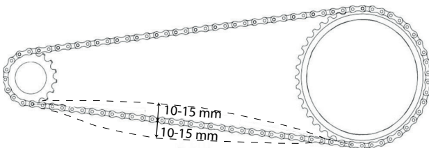
Abbildung 126: Kettenspannung prüfen
