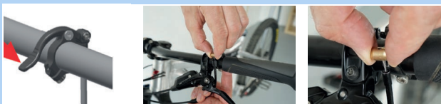
Abbildung 136: Kartusche Ausbauen
