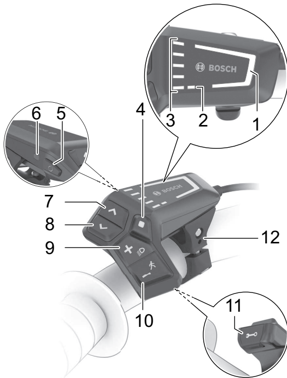
Abbildung 105: Übersicht Bedieneinheit BOSCH LCD Remote
