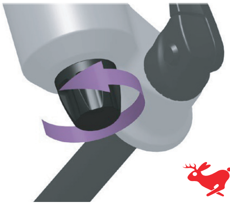
Abbildung 207: Zugstufen-Schraube in Richtung Hase drehen
