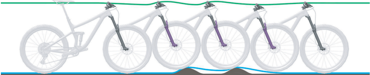
Abbildung 206: Zu langsames Ausfedern der Federgabel
